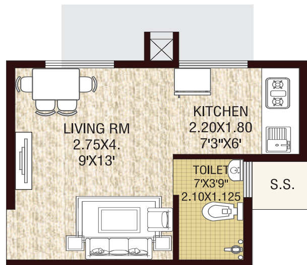
UNIT TYPE - 1RK WING- E3 & E4
