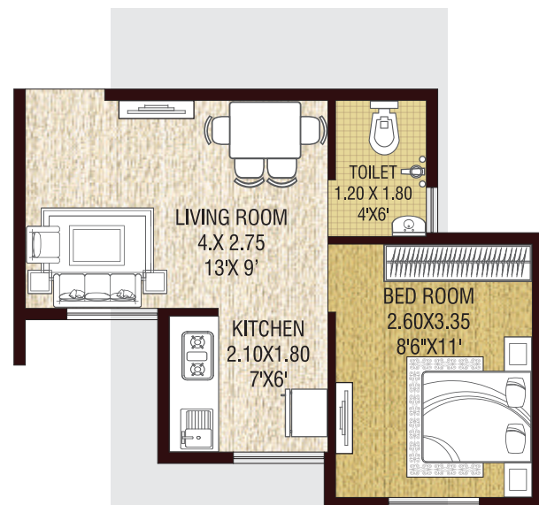
WING-E2,E7,E11 & E12 UNIT TYPE - 1BHK
